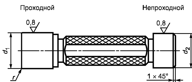
Рисунок А.2 — Проходные и непроходные калибры-пробки для контроля охватываемых концов фитингов
