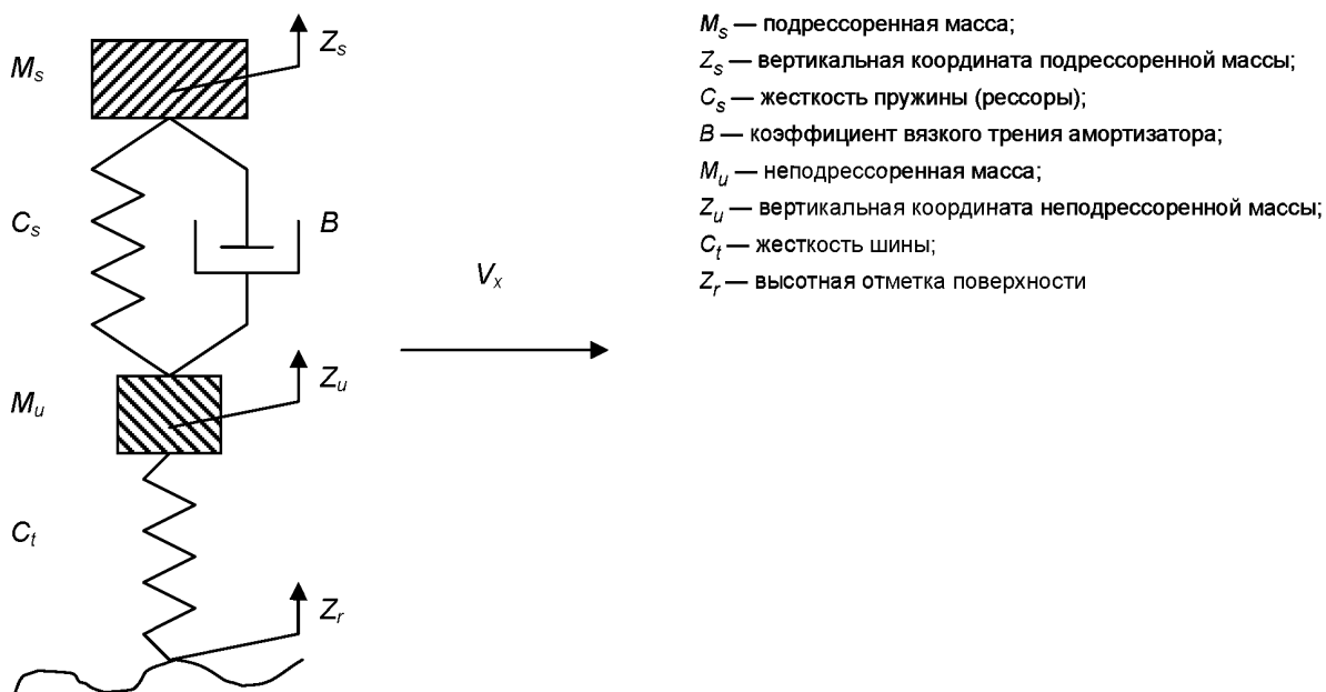
Рисунок В.1 — Модель автомобиля для расчета IRI
