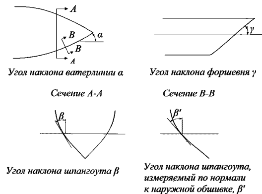
Рис. 1.2.3.2.1.1.1 Определение углов наклона
