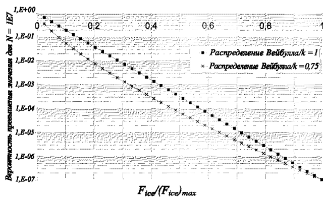
Рис.10.7.5.1.8 Распределение Вейбулла
