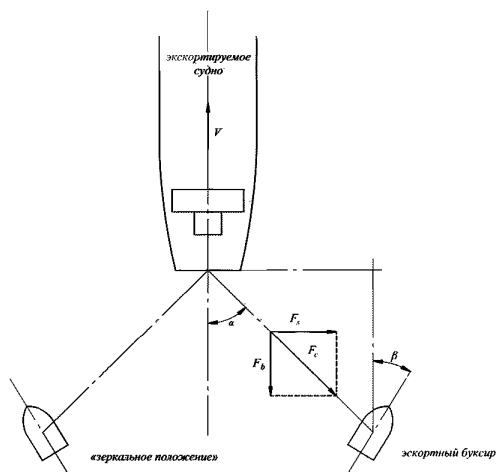
Рис. 2.1.2 Типовая схема эскортных операций: F_s — удерживающая сила; F_b — тормозящая сила; F_t — натяжение буксирного троса; \alpha — угол отклонения буксирного троса эскортного буксира от диаметральной плоскости эскортируемого судна; \beta — угол отклонения курса эскортного буксира от курса эскортируемого судна; V — скорость эскортируемого судна
