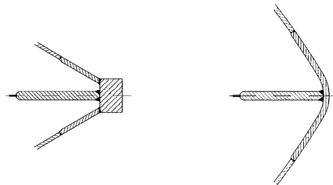
Рис. 10.5.7.1 Примеры допустимой конструкции форштевня
