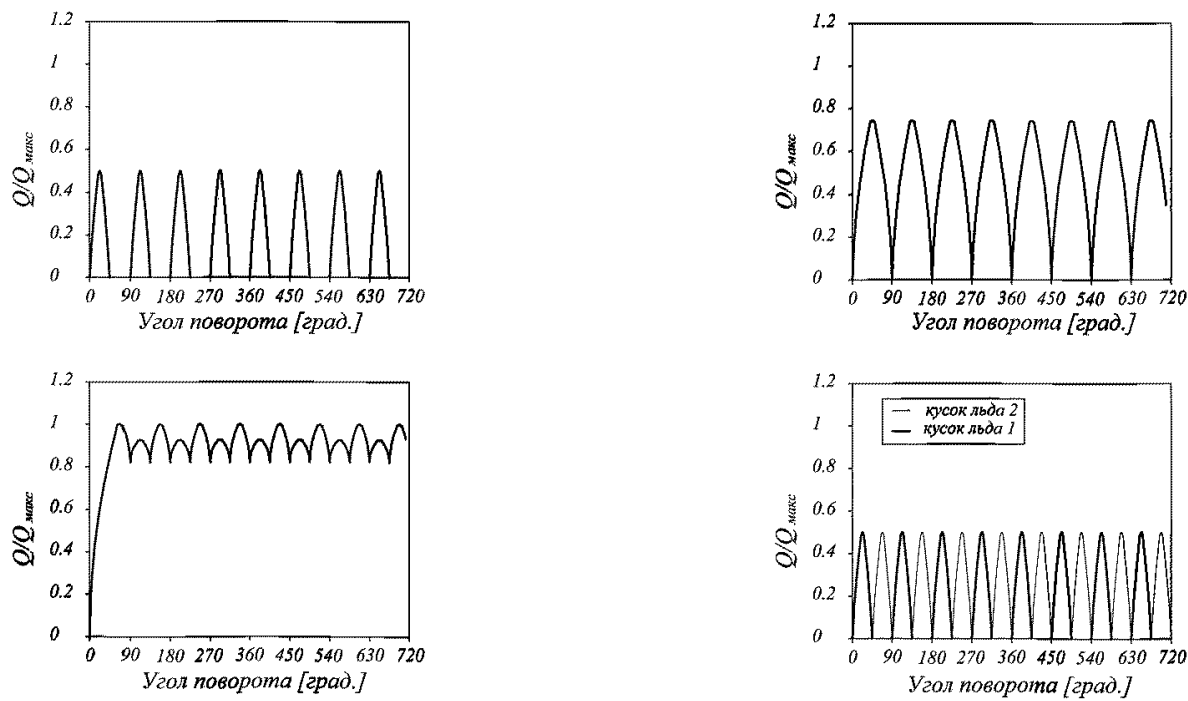
Рис. 1 Процесс изменения ледового момента сопротивления вращению гребного винта (крутящий момент на гребном винте) для последовательности 45, 90, 135° столкновения единичной лопасти и 45° двойной последовательности столкновения лопасти (два куска льда) для 4-лопастного винта
