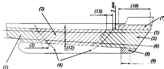
Рис. 10.5.1.1 Районы ледовых усилений корпуса судна:
