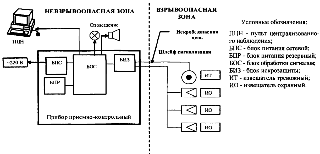
Рис.6.2 Оборудование объекта с взрывоопасными зонами.
