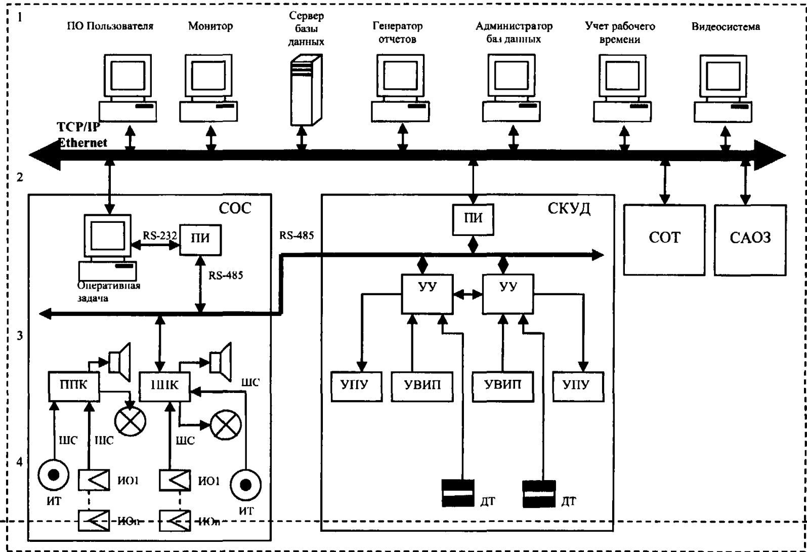
Рис. 2.1. Обобщенная структура ИСБ на основе локальных сетей.
