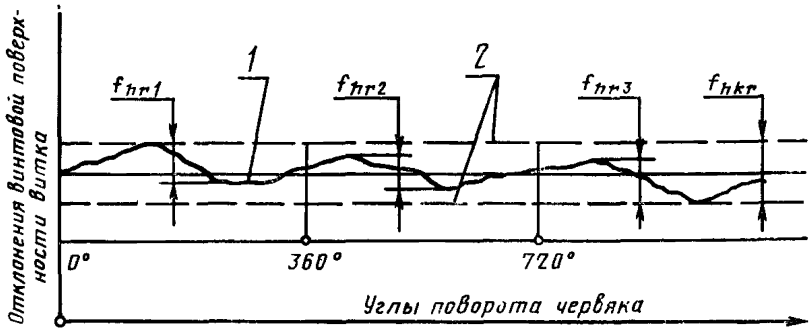
1—действительная винтовая линия; 2—номинальные винтовые линии
