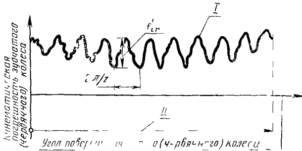
I—кривая кинематической погрешности червячного колеса; II—одни оборот червячного колеса
