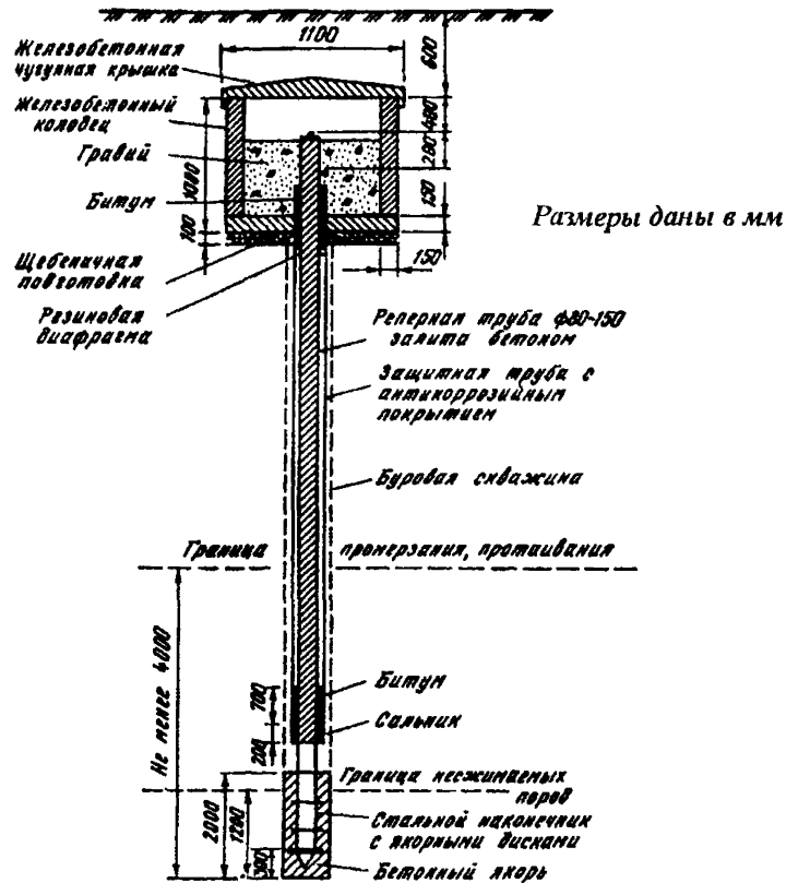
Рис.2 Вековой трубчатый репер. Тип 175 к
