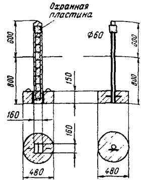
Рис. 16 Опознавательные столбы для области сезонного промерзания грунтов
