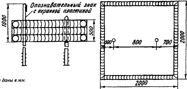
Рис. 19 внешнее оформление реперов в области многолетней мерзлоты
