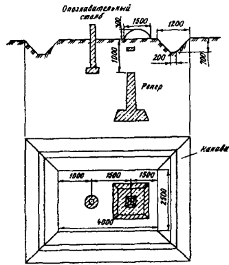
Рис. 15 Внешнее оформление фундаментальных реперов в области сезонного промерзания грунтов
