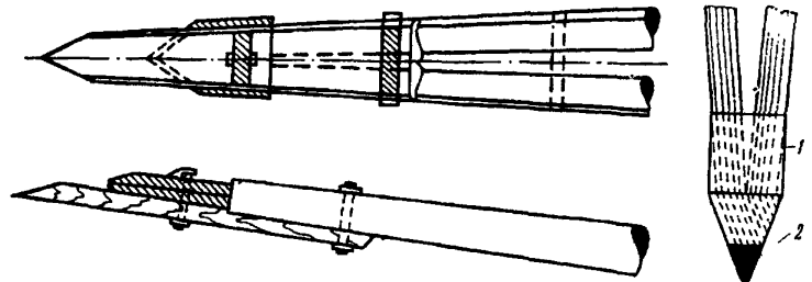
Рис. 26 Текстолитовый (деревянный) удлинитель
