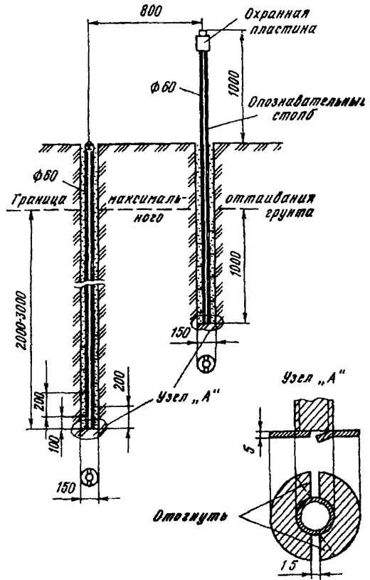
Рис. 9. Грунтовый репер для области многолетней мерзлоты. Тип 150 оп. зна
