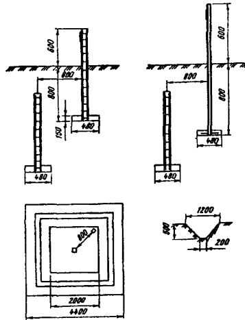
Рис. 18 Внешнее оформление грунтового репера
