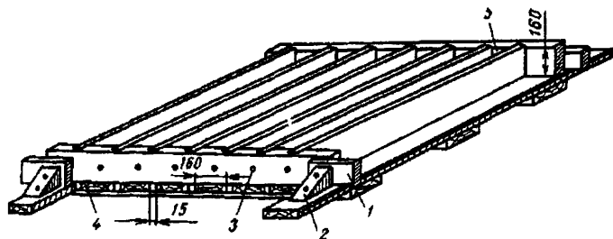
Рис. 28 Многоячейковая опалубка:
