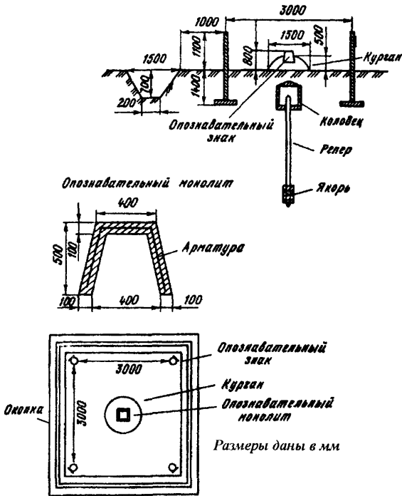
Рис. 14. Внешнее оформление вековых реперов
