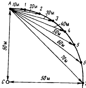
Рис.30 Схема размещения нивелира и рейки
