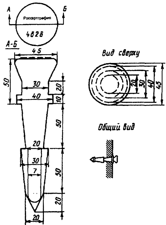
Рис.12. Стеной репер для линий нивелирования I и II классов Тип 143
