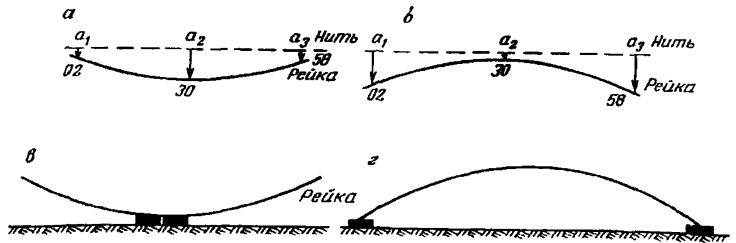
Рис. 32. Схемы определения стрелки прогиба рейки
