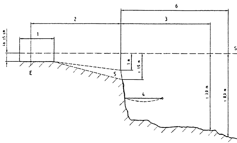
Рисунок 1. Зоны посадки на кресельных КД
