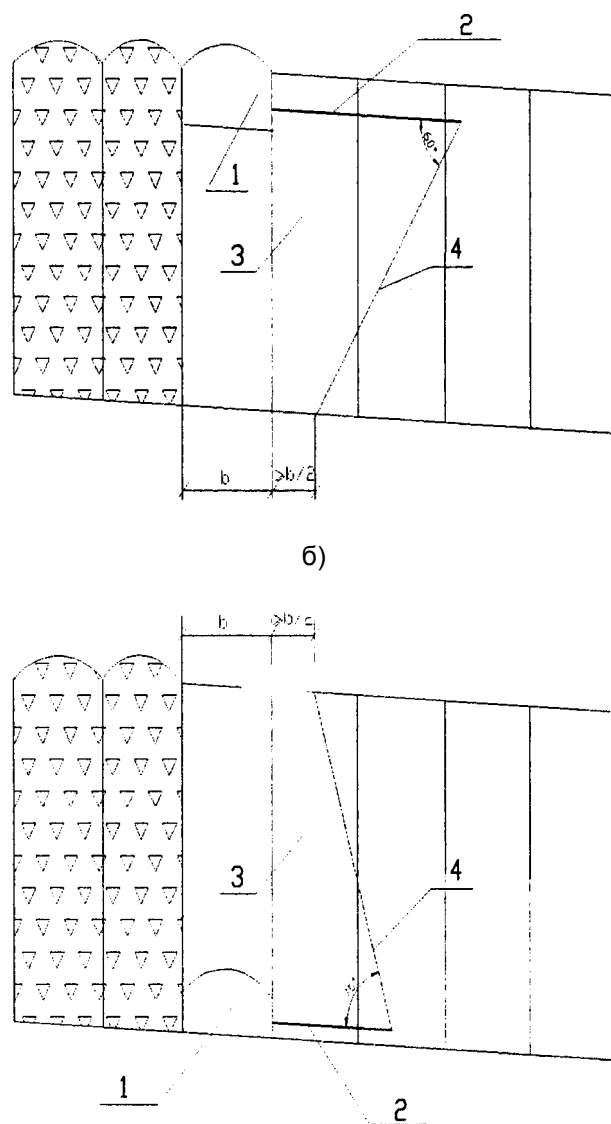
Рисунок 5 - Построение защищенной зоны бурением скважин большого диаметра по кровле (а) и почве (б) рудного тела 1 - выработка; 2 - скважина; 3 - защищенная зона; 4 - граница защищенной зоны; b - ширина ленты
