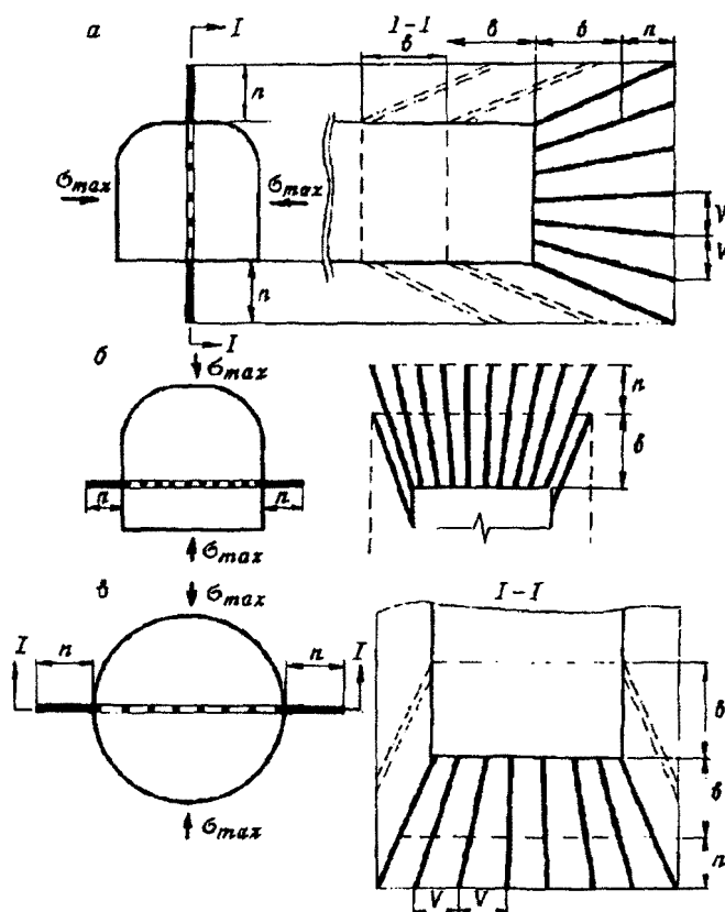
Рисунок 11 - Схемы камуфлетного взрывания по рядам шпуров:
