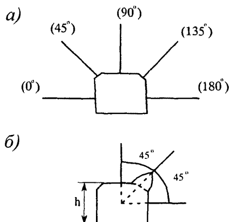
Рисунок 8 - Типовые схемы замерных станций для определения категории удароопасности выработки: а - при равномерном разрушении контура выработки; б - при хорошо выраженном месте максимального разрушения контура
