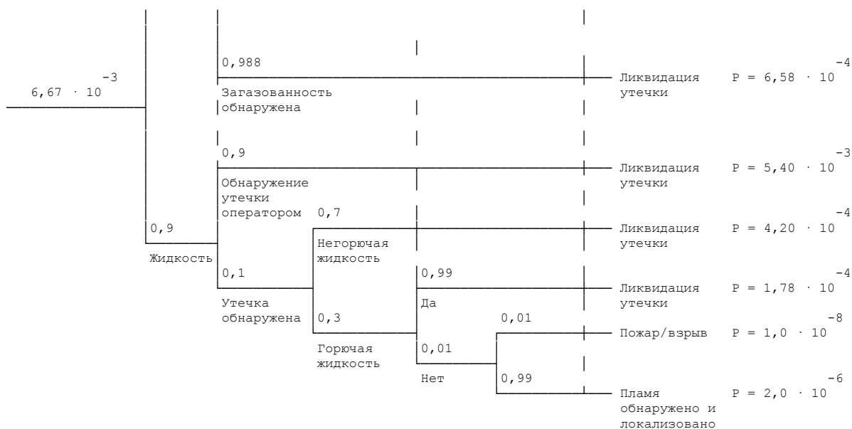
Рис. 8-2. Пример дерева событий для случая разгерметизации сосудов, работающих под давлением
