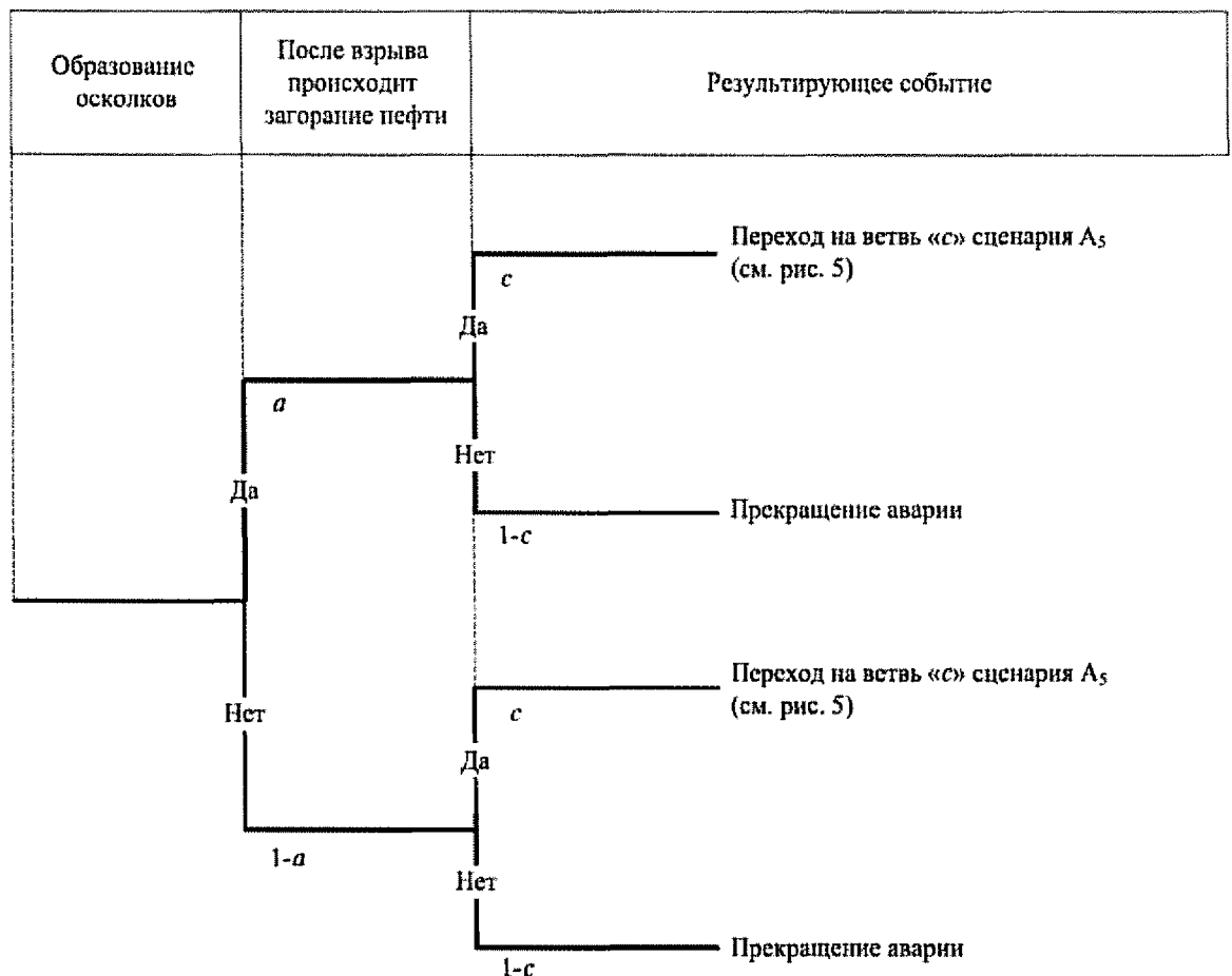
Рис. 6. «Дерево событий» при взрыве внутри подземного резервуара (типа ЖБР) (сценарий А 6 )
